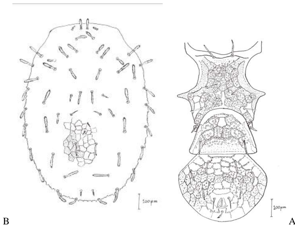
شکل ۱- سطح شکمی (A) و سطح پشتی (B) کنه ماده Glyptholaspis confuse (شکل اصلی)
