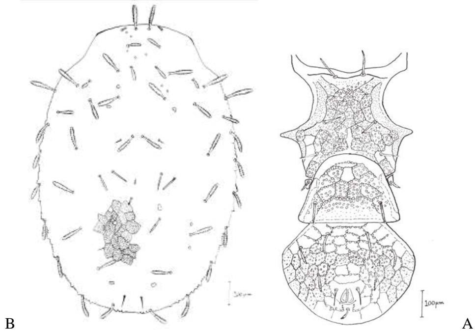
شکل ۲- سطح شکمی (الف) و سطح پشتی (ب) کنه ماده Glyphtholaspis sp. (شکل اصلی) Figure 2. Female Glyphtholaspis sp., ventral (A) and dorsal (B) view (Original)
