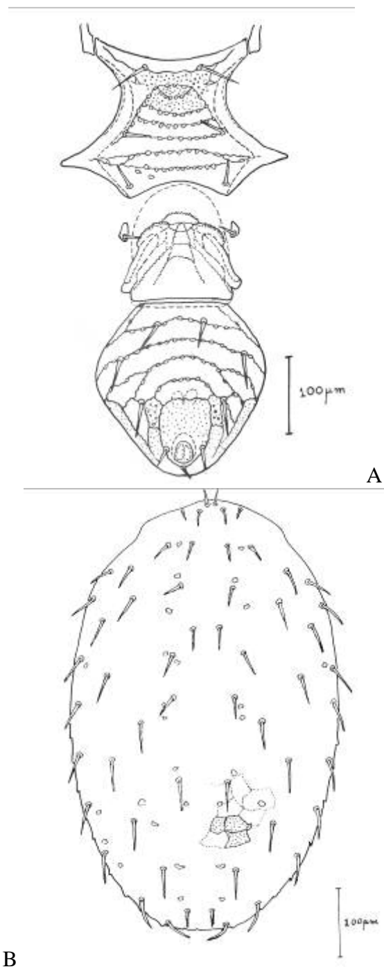
شکل ۴- سطح شکمی (الف) و سطح پشتی (ب) کنه ماده Macrocheles subbadius (شکل اصلی)
