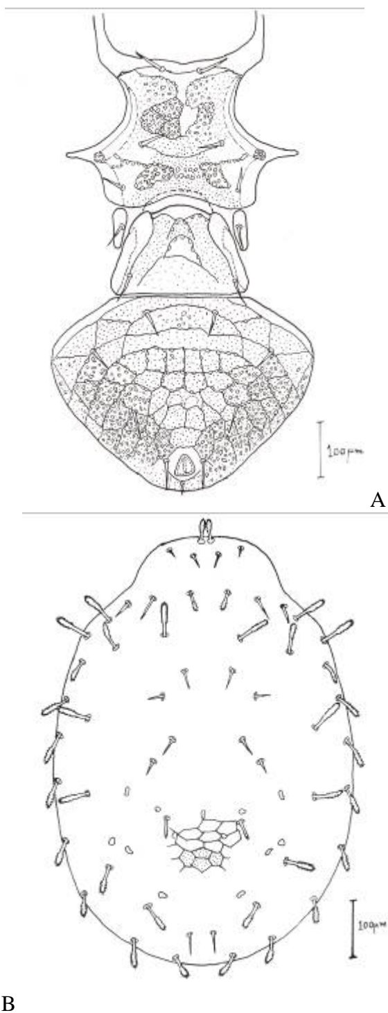
شکل ۵- سطح شکمی (الف) و سطح پشتی (ب) کنه ماده Macrocheles peniculatus (شکل اصلی) Figure 5. Female Macrocheles peniculatus , ventral (A) and dorsal (B) view (Original)
