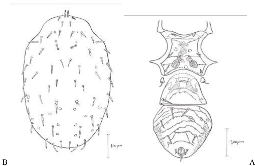
شکل ۱۱- سطح شکمی (الف) و سطح پشتی (ب) کنه ماده 1 Macrocheles sp. (شکل اصلی)
