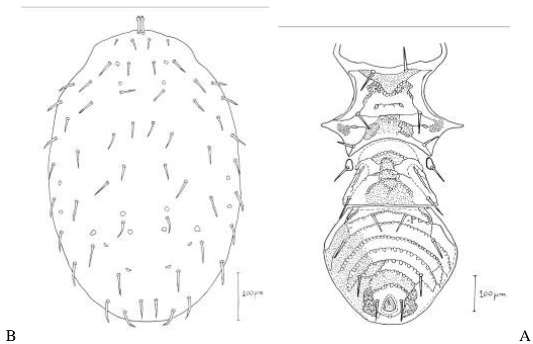
شکل ۹- سطح شکمی (الف) و سطح پشتی (ب) کنه ماده Macrocheles sp. 2 (شکل اصلی) Figure 9. Female Macrocheles sp. 2, ventral (A) and dorsal (B) view (Original)
