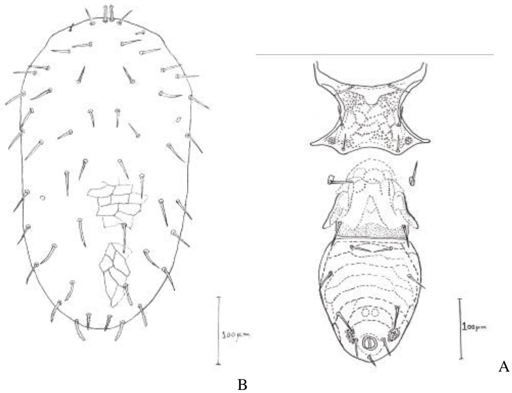
شکل ۱۰- سطح شکمی (الف) و سطح پشتی (ب) کنه ماده 3 Macrocheles sp. (شکل اصلی)
